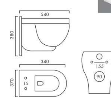
KWID Design No.: 2002
