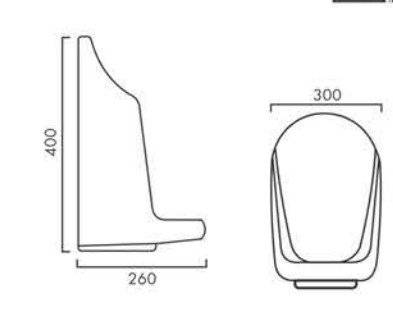
MINI LARGE URINAL Design No.: 7053
